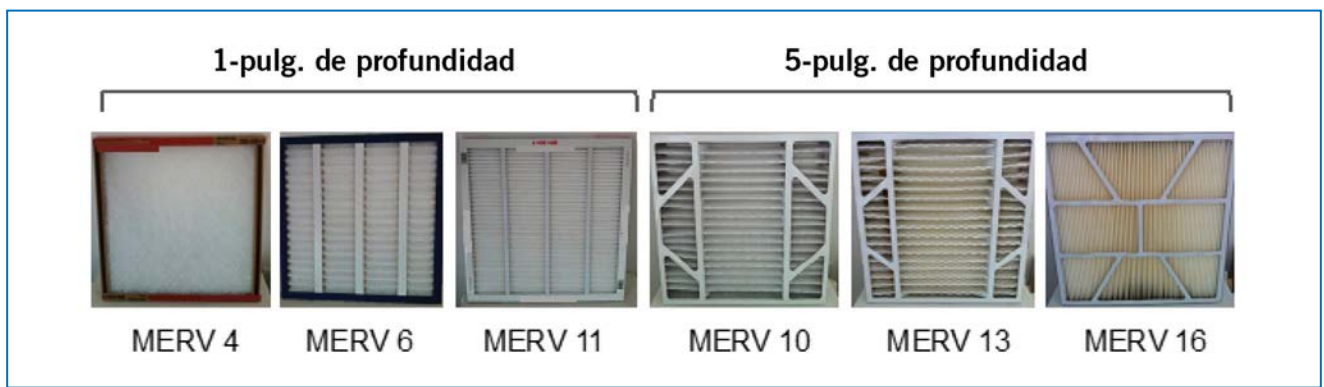
Figura 4. Ejemplos de varios filtros de medios de materiales fibrosos instalados en ductos para aplicaciones residenciales de aire central disponibles en el mercado. Imagen cortesía de Brent Stephens.
