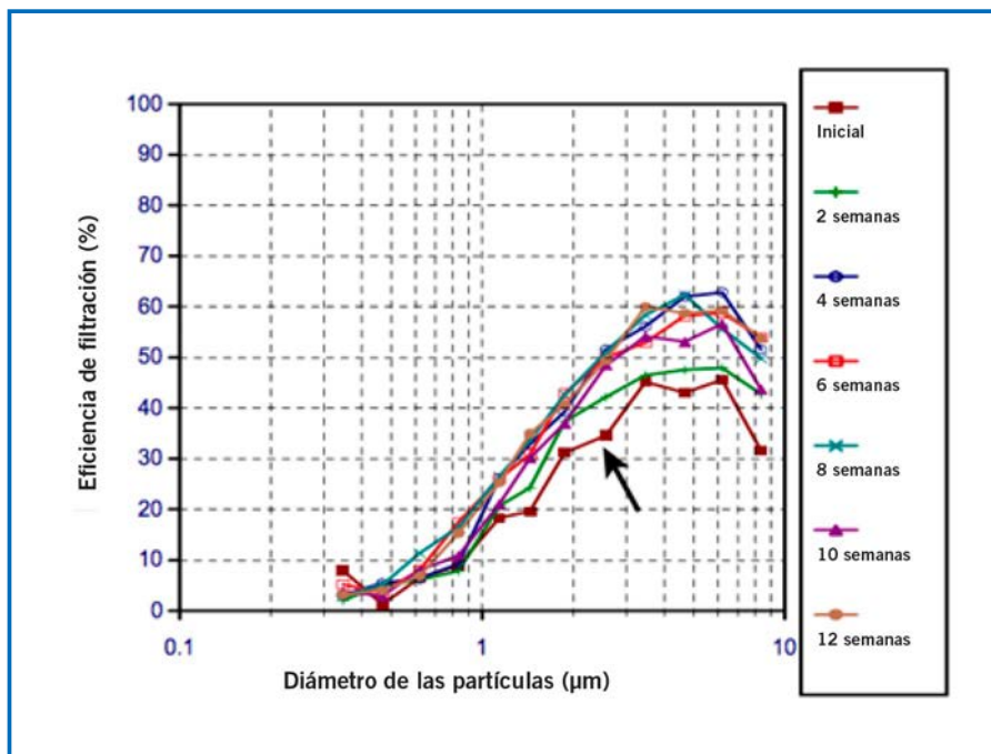
Figura 6. Ejemplo de curvas de eficiencia de eliminación resuelta por tamaño para filtros de aire de medios de material fibroso nuevos (MERV 5 cuando están limpios) y filtros de aire cargados, que no sean electret, de medios de materiales fibrosos como lo indican los ensayos reportados en Hanley and Owen (2003). ©ASHRAE del ASHRAE Research Project Final Report 1190-RP.
